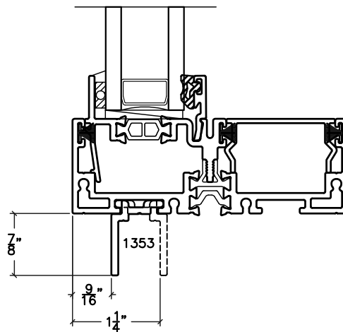
NAIL FIN OPTIONS
