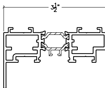
3500 STD. FRAME
