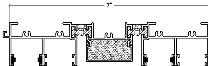
A7 ACOUSTIC FRAME
